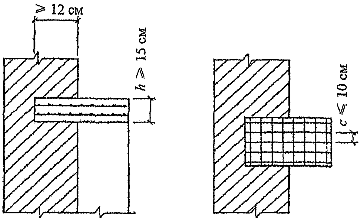
Рисунок 13 – Железобетонные распределительные плиты
