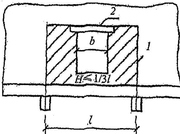
Рисунок 17 – Схема нагрузки на рандбалку при наличии проема в стене Карнизы и парапеты
