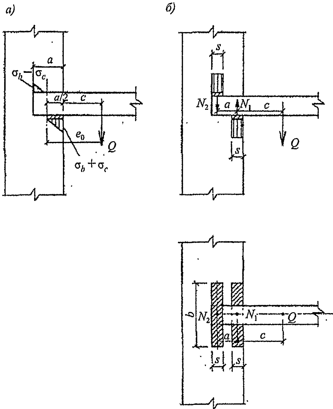
Рисунок 14 – Расчетные схемы заделки консольных балок
