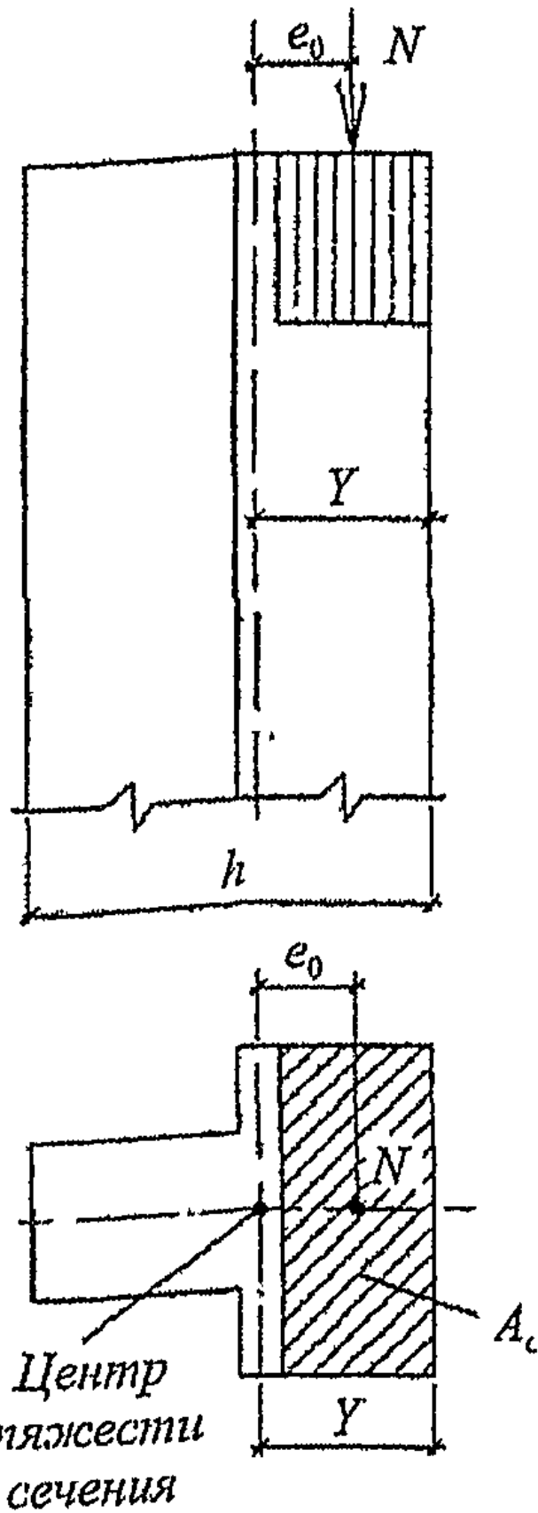
Рисунок 5 – Внецентренное сжатие
