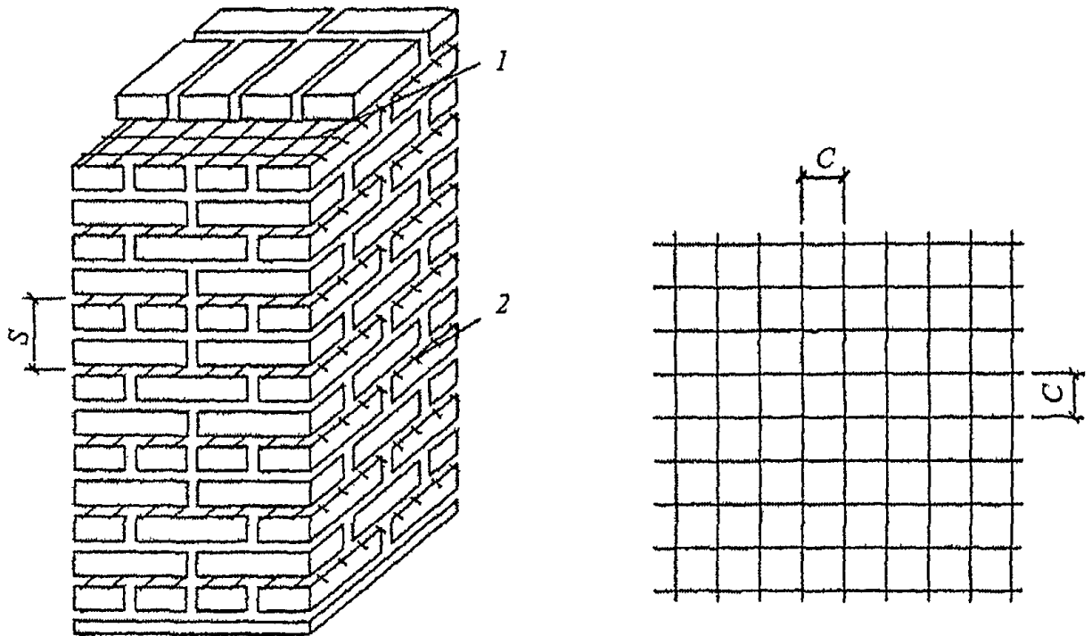
Рисунок 11 – Поперечное (сетчатое) армирование каменных конструкций
