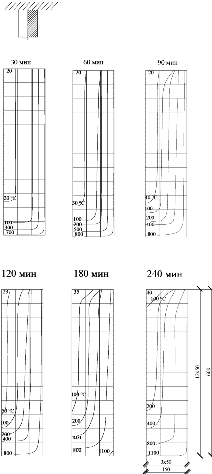
Рисунок И.10 - Балка из легкого бетона сечением 600x300 мм при нагреве с трех сторон
